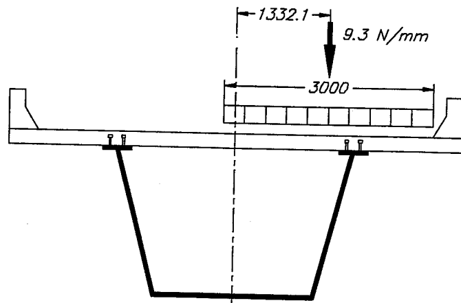
a) Lane Load
