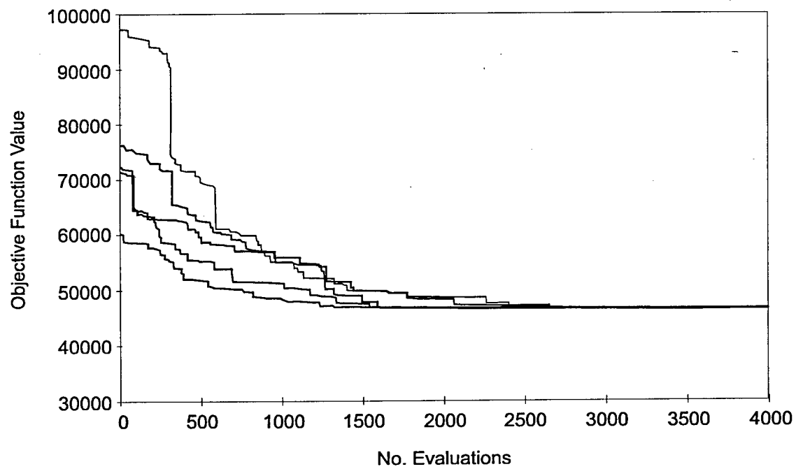
Figure 17. SA Results for Case 2
