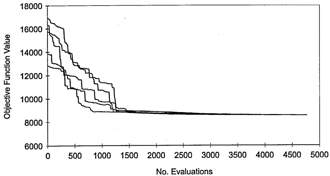
Figure 16. SA Results for Case 1
