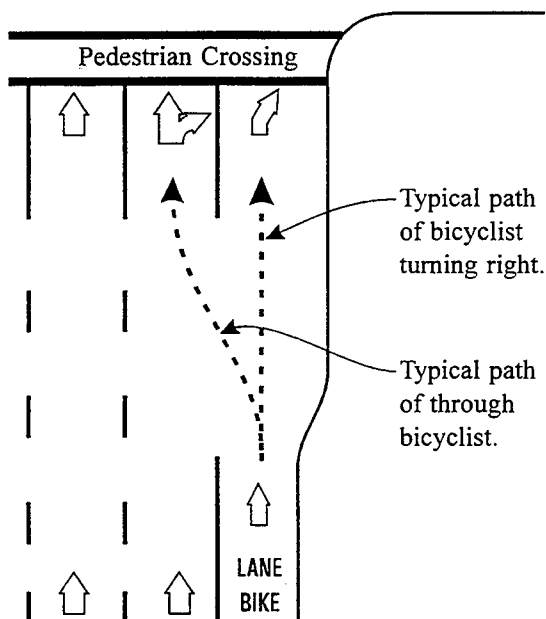
(3) Optional double right-turn-only lane
