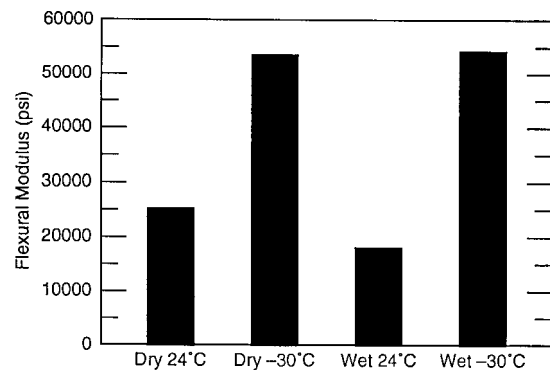
b. Flexural modulus.
