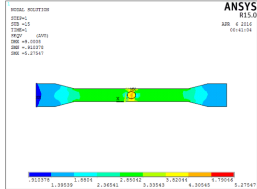
NS_0.3 von Mises stress
